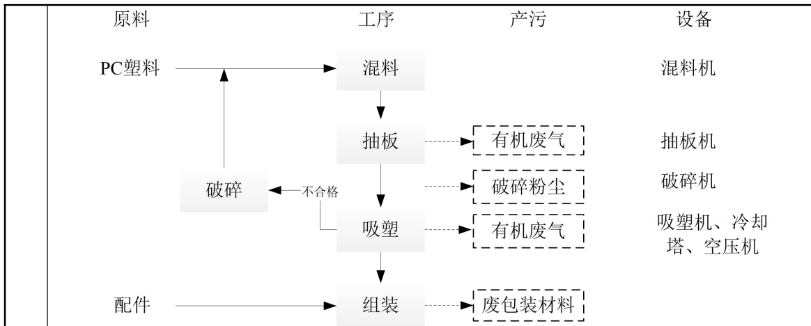
图 2-3 PC 箱生产工艺流程图
