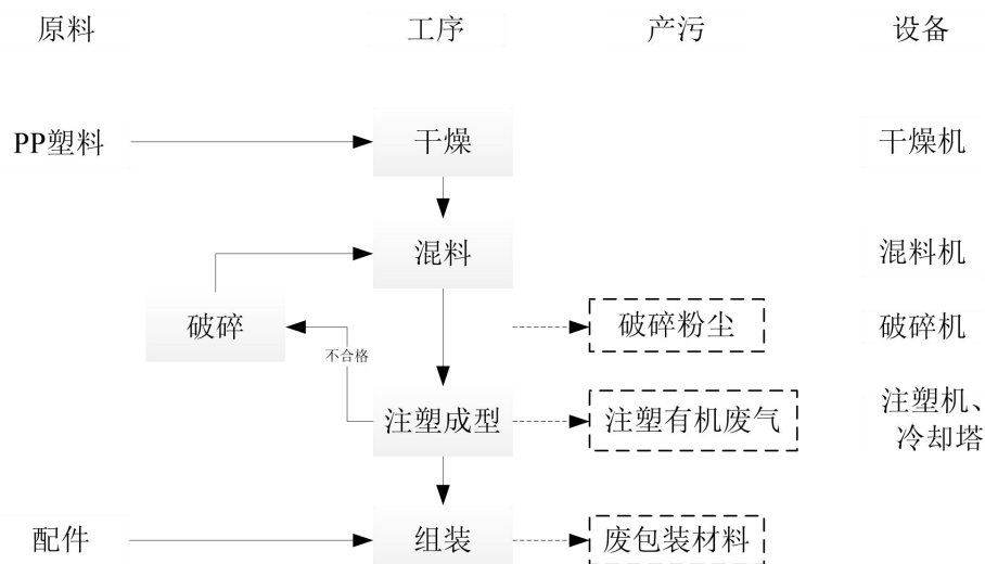
图 2-2 PP 箱生产工艺流程图
