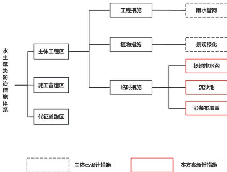
图 5.2-1 防治措施体系框图
