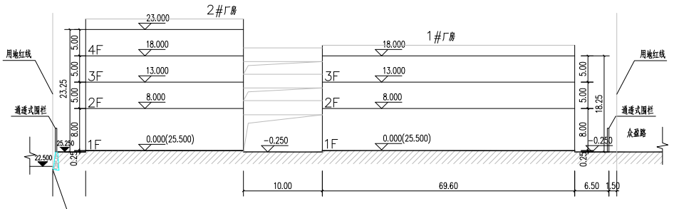
1-1剖面示意图 1:500
