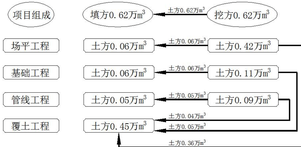
图 1.3-1 土石方流向框图 单位：万 m 3
