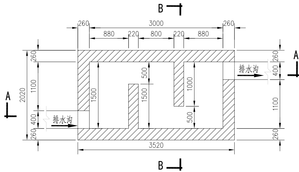
沉沙池平面图 1:50
