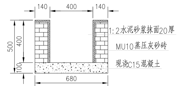
场地排水沟大样图 1:20
