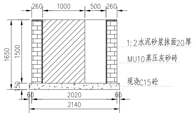
B-B断面图 1:50
