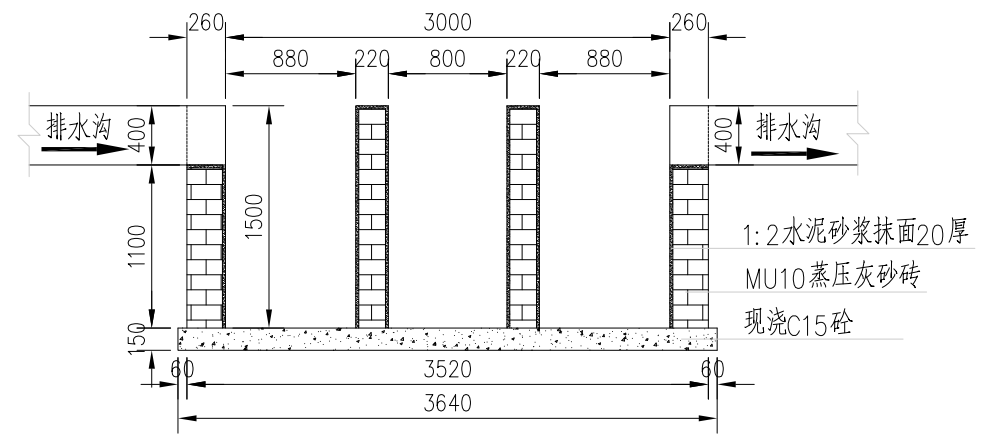
A-A断面图 1:50
